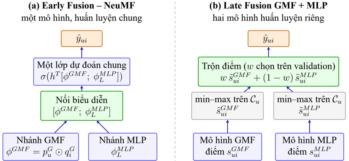
Hình 2.2: Hai cách hợp nhất cùng hai thành phần MF (GMF) và DNN (MLP): ở mức biểu diễn (NeuMF) và ở mức điểm dự đoán (Late Fusion)
