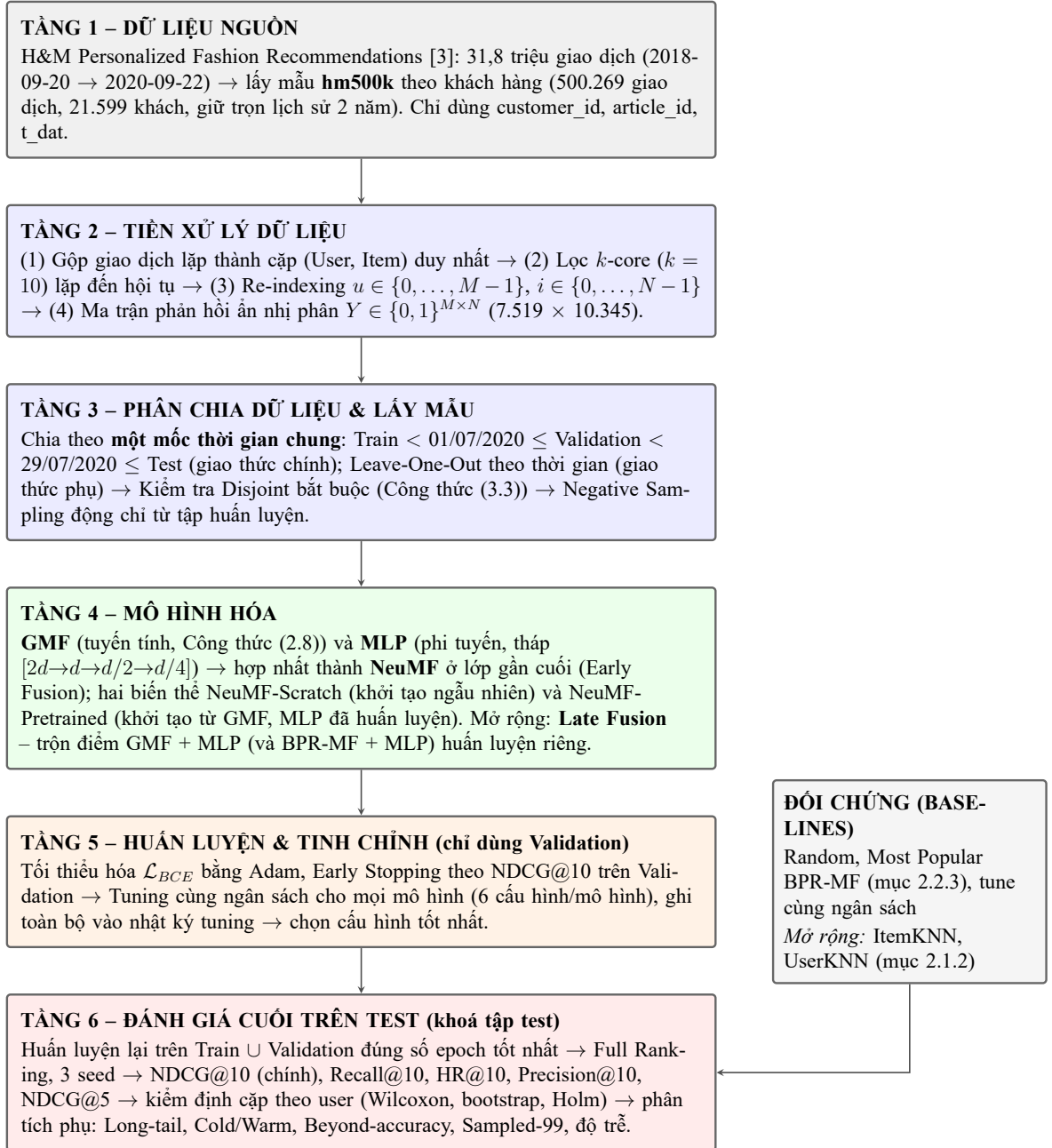
Hình 3.1: Kiến trúc tổng thể của hệ thống nghiên cứu, từ dữ liệu thô H&M đến đánh giá cuối trên tập test
