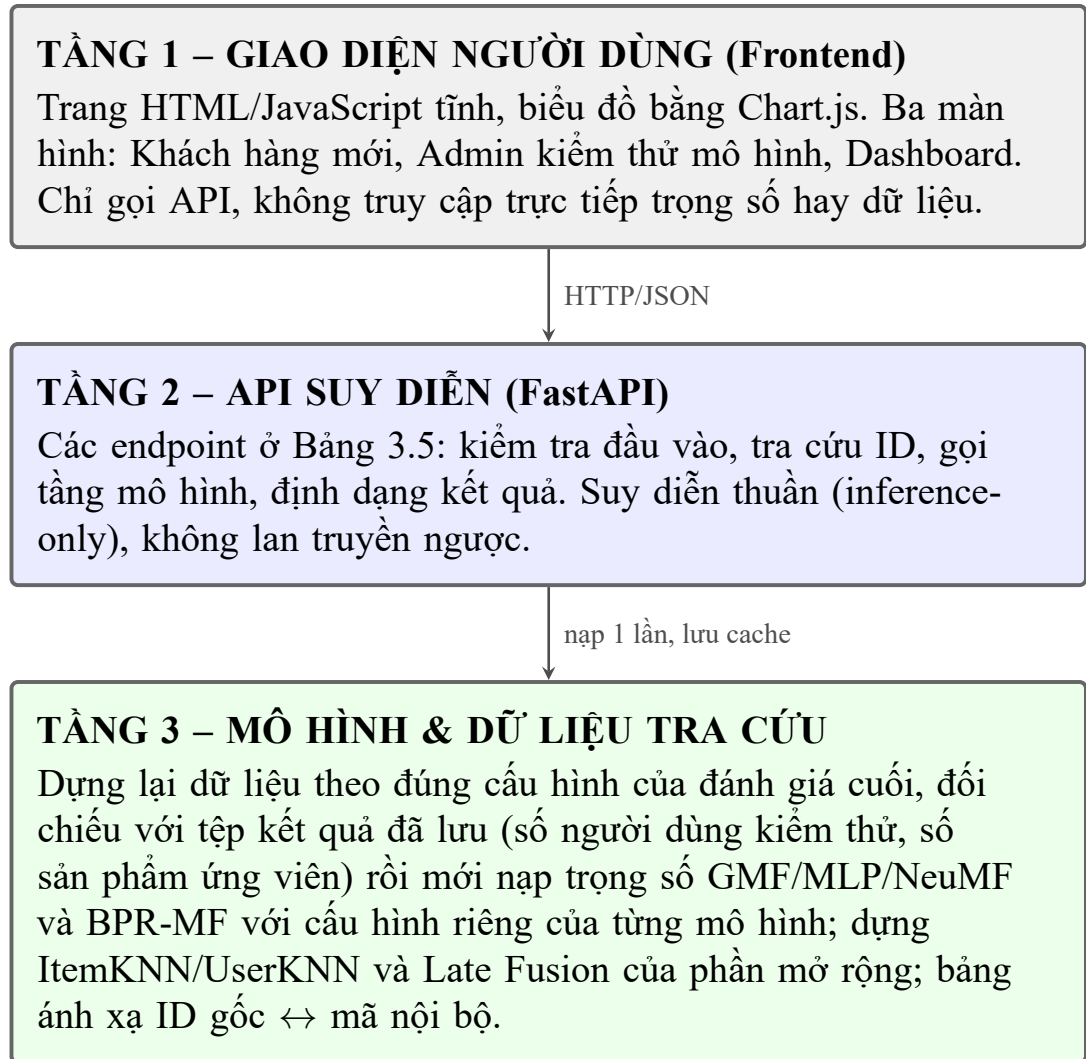
Hình 3.2: Kiến trúc ba tầng của hệ thống giao diện thực nghiệm (demo)
